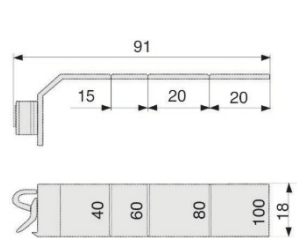
TR1 Wire retaining clip
