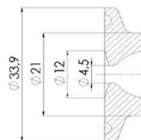
Mini flange
