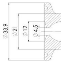
Mini flange
