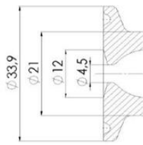
Mini flange
