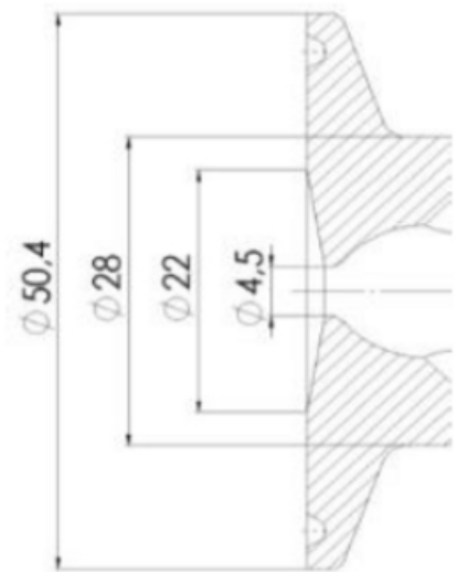
Clamp Ø 50,4
