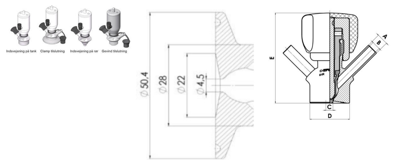
Clamp Ø 50,4
