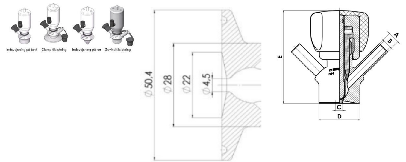
Clamp \varnothing 50,4
