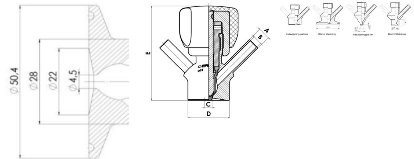
Clamp \varnothing 50,4
