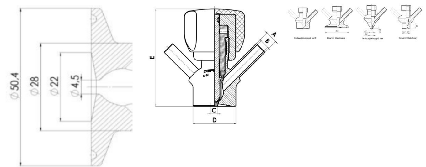
Clamp Ø 50,4
