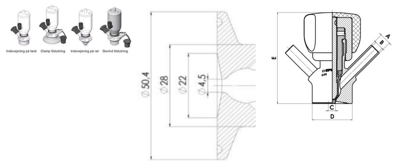
Clamp Ø 50,4
