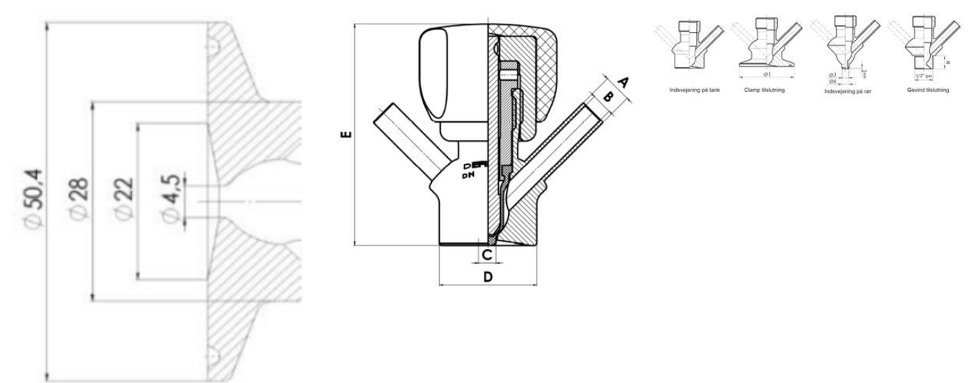
Clamp Ø 50,4
