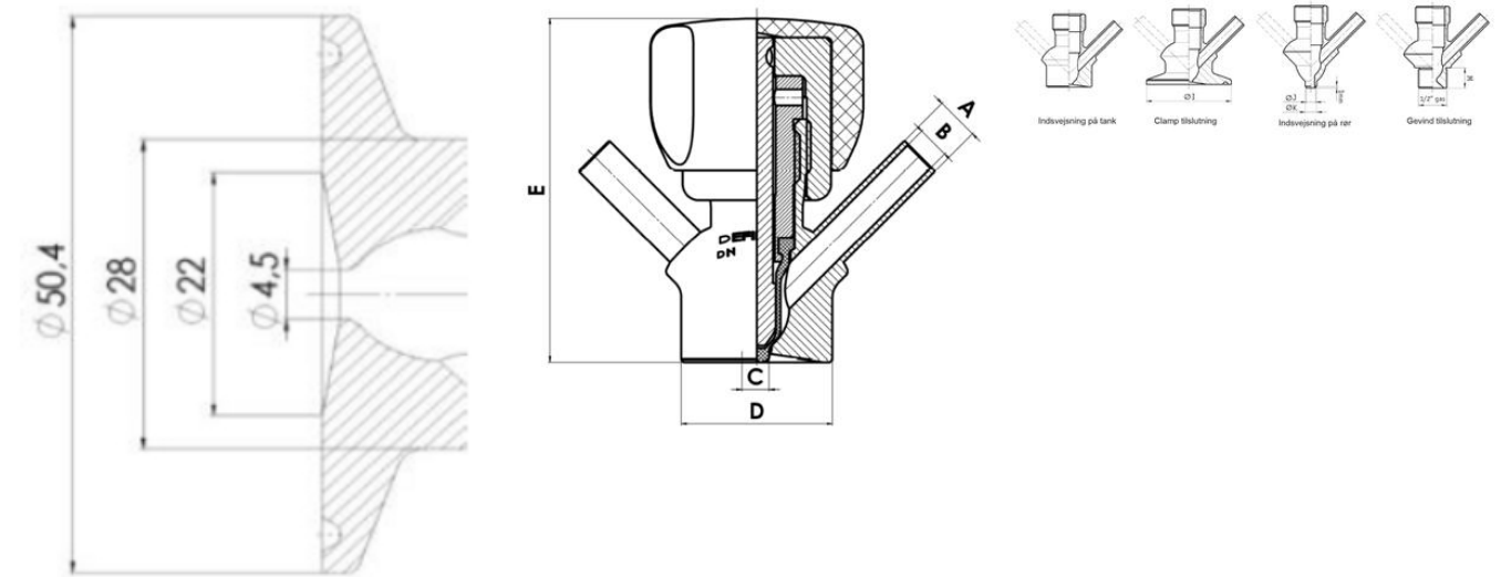
Clamp Ø 50,4
