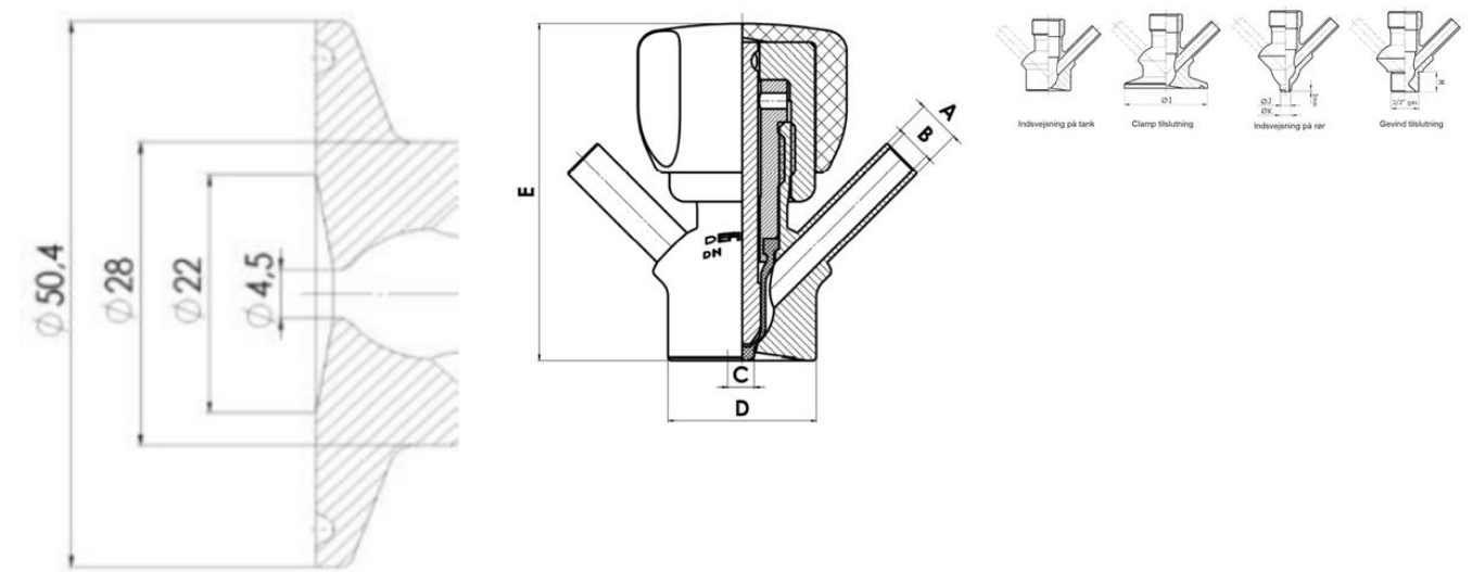
Clamp Ø 50,4
